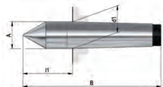
A07 DIN 806, full point, material: tool steel
